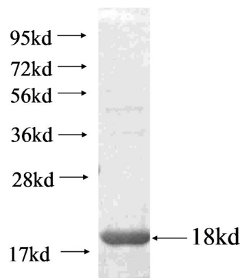
Recombinant Arabidopsis thaliana EDF1 SDS-PAGE
