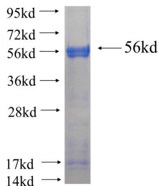
Recombinant Arabidopsis thaliana PKT3 SDS-PAGE
