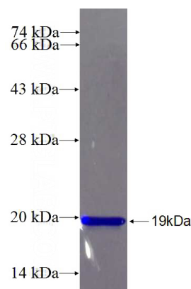
Recombinant Human ADAM22 SDS-PAGE
