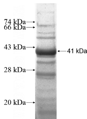
Recombinant Human SH3BP4 SDS-PAGE
