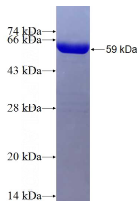
Recombinant Human ACTN4 SDS-PAGE
