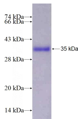
Recombinant Human TTK SDS-PAGE
