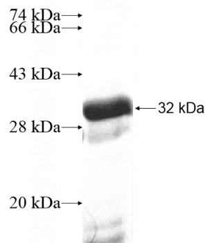
Recombinant Human GPR176 SDS-PAGE
