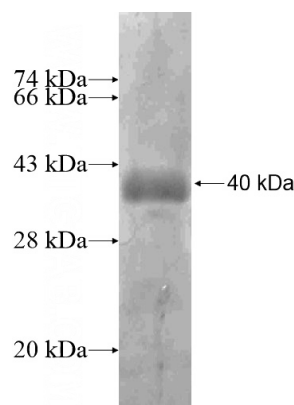
Recombinant Human C10orf119 SDS-PAGE
