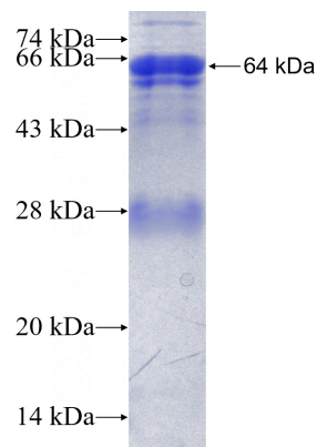
Recombinant Human EHD2 SDS-PAGE
