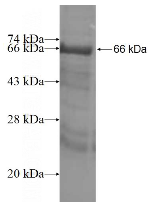
Recombinant Human SRP54 SDS-PAGE
