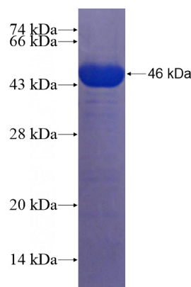
Recombinant Human ZBTB46 SDS-PAGE
