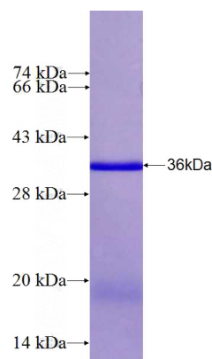
Recombinant Human TRAFD1 SDS-PAGE
