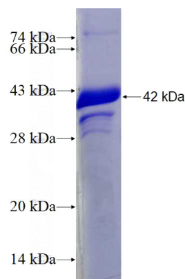
Recombinant Human BMP-7 SDS-PAGE
