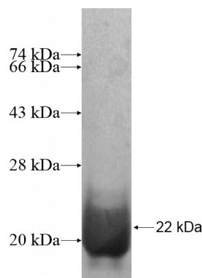
Recombinant Human TAF10 SDS-PAGE
