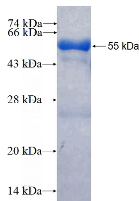
Recombinant Human RARRES1 SDS-PAGE
