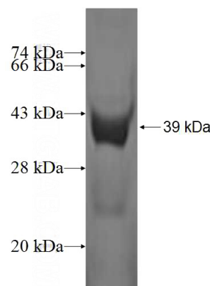
Recombinant Human SH3BGRL SDS-PAGE
