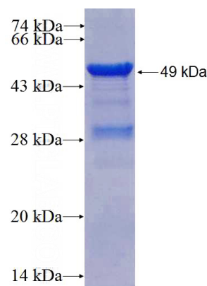
Recombinant Human RALB SDS-PAGE
