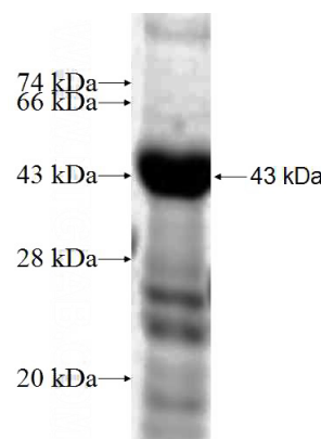
Recombinant Human NPHP4 SDS-PAGE
