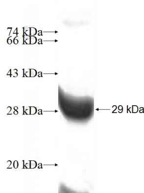
Recombinant Human POP4 SDS-PAGE
