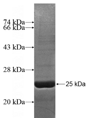
Recombinant Human C14orf143 SDS-PAGE
