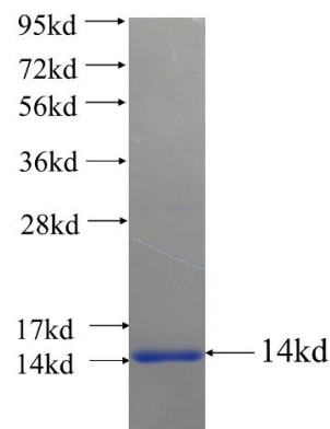
Recombinant human TMIE SDS-PAGE
