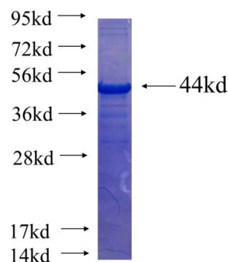
Recombinant human NLRX1 SDS-PAGE
