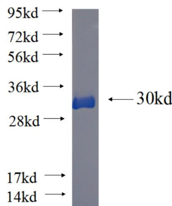
Recombinant human KIF5C SDS-PAGE
