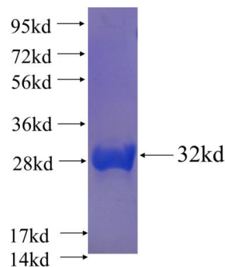
Recombinant human HOXA13 SDS-PAGE
