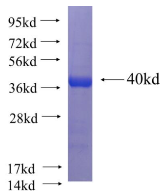
Recombinant human HDAC1 SDS-PAGE
