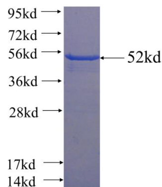
Recombinant human CLNS1A SDS-PAGE
