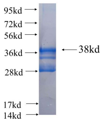
Recombinant human C20orf149 SDS-PAGE
