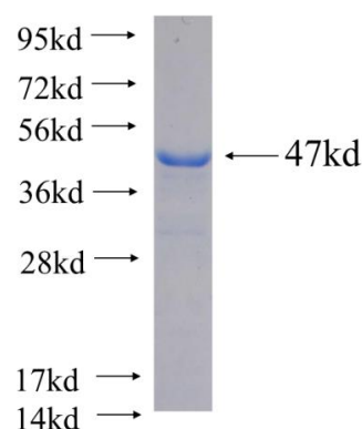
Recombinant human ABCD2 SDS-PAGE
