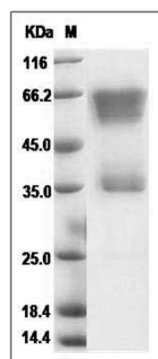
Cynomolgus EDAR Protein (Fc Tag) SDS-PAGE
