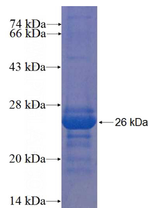
Recombinant Human KIAA0247 SDS-PAGE
