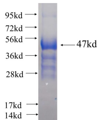
Recombinant human NANOS3 SDS-PAGE
