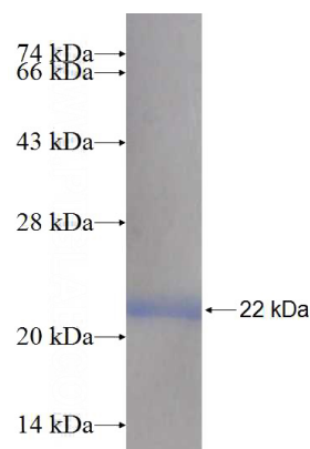
Recombinant Human CETN3 SDS-PAGE
