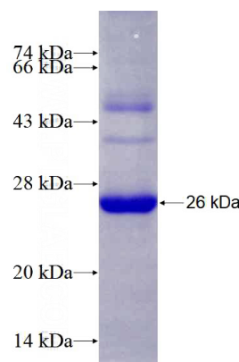
Recombinant Human ABCE1 SDS-PAGE
